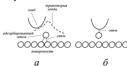
Рисунок 1.6 – Иллюстрация траектории острия зонда СТМ
