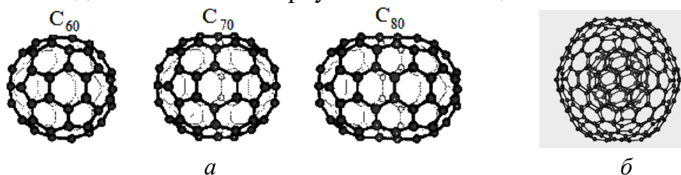
Рисунок 1.22 –Примеры структур на основе углеродных кластеров: а – фуллерены C_{60} , C_{70} , C_{80} ; б – многослойный фуллерен C_{60}/C_{240}
