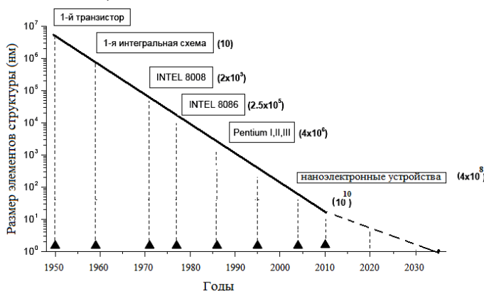
Рисунок 1.30 – Динамика уменьшения размеров элементов интегральных схем (в скобках указано число транзисторов)
