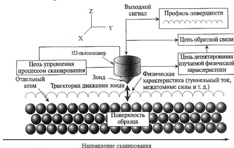
Рисунок 1.2 – Типовая схема зондовых сканирующих микроскопов
