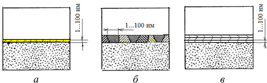
Рисунок 1.9 – Наноструктурные покрытия: а – нанослойные; б – нанокристаллические; в – многослойные
