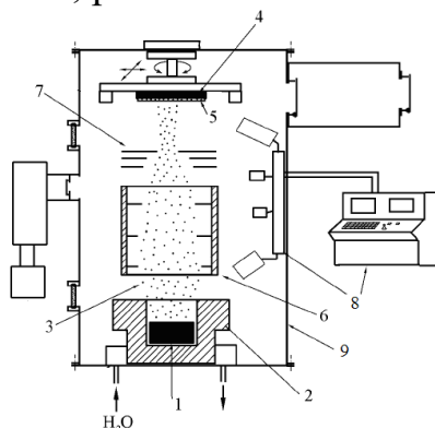
Рисунок 1.28 – Типичная схема установки для нанесения покрытия PVD -методом:
