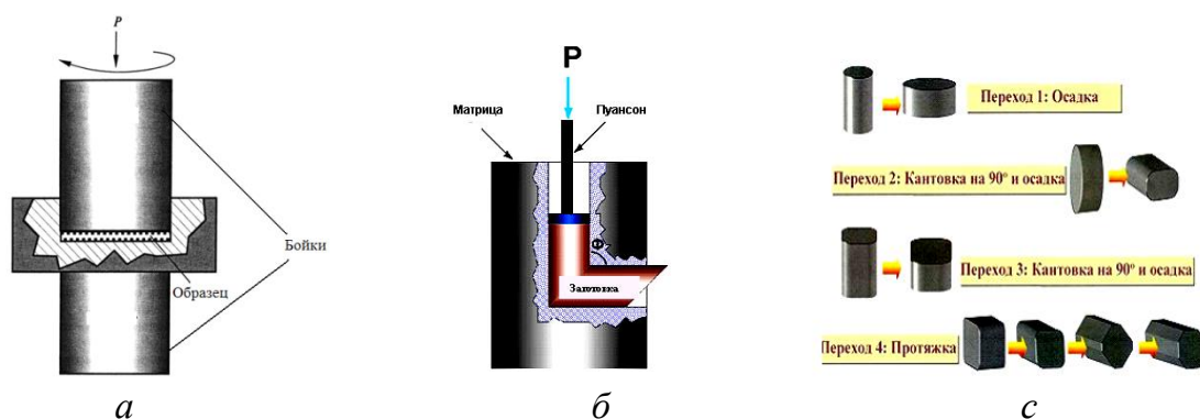
Рисунок 1.26 – Основные методы ИПД: a – кручение под давлением; б – равноканальное угловое прессование; в - всесторонняя ковка
