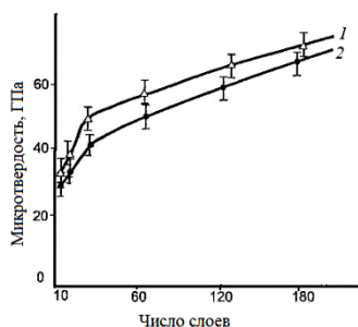
Рисунок 1.29 – Зависимость микротвердости многослойных покрытий толщиной 2 \pm 0,3 мкм TiN/NbN (1), TiN/ZrN (2) от количества слоев в покрытии (толщины слоя)
