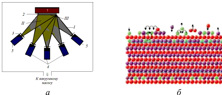
Рисунок 1.10 – Схема установки молекулярно-лучевой эпитаксии ( а ) и схема роста пленки путем «атомной укладки» ( б ):
