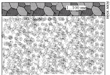
Рисунок 1.27 – Нанокристаллическое покрытие
