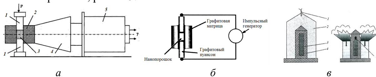
Рисунок 1.25 – Схемы методов динамического прессования: а – установка для ультразвукового прессования: 1 – пуансон; 2 – матрица; 3 – заготовка; 4 – УЗ-концентратор; 5 – магнестрикционный преобразователь, соединенный с УЗ-генератором; б – агломерация пульсирующим электрическим током; в – схема взрывного компактирования: 1 – электродетонатор; 2 – заряд взрывчатого вещества; 3 – прессуемый порошок; 4 – ампула; 5 – спрессованный порошок (компакт)
