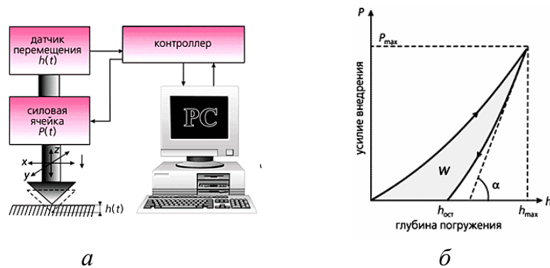
Рисунок 1.3 – Принципиальная схема нанотестирования поверхности (а) и типичная диаграмма «сила-перемещение» при наноиндентировании – аналог диаграммы \sigma - \varepsilon в традиционных макроиспытаниях (б): h_{max} – максимальная глубина внедрения индентора; h_{ост} – глубина отпечатка, оставшегося после снятия нагрузки; W – поглощенная энергия
