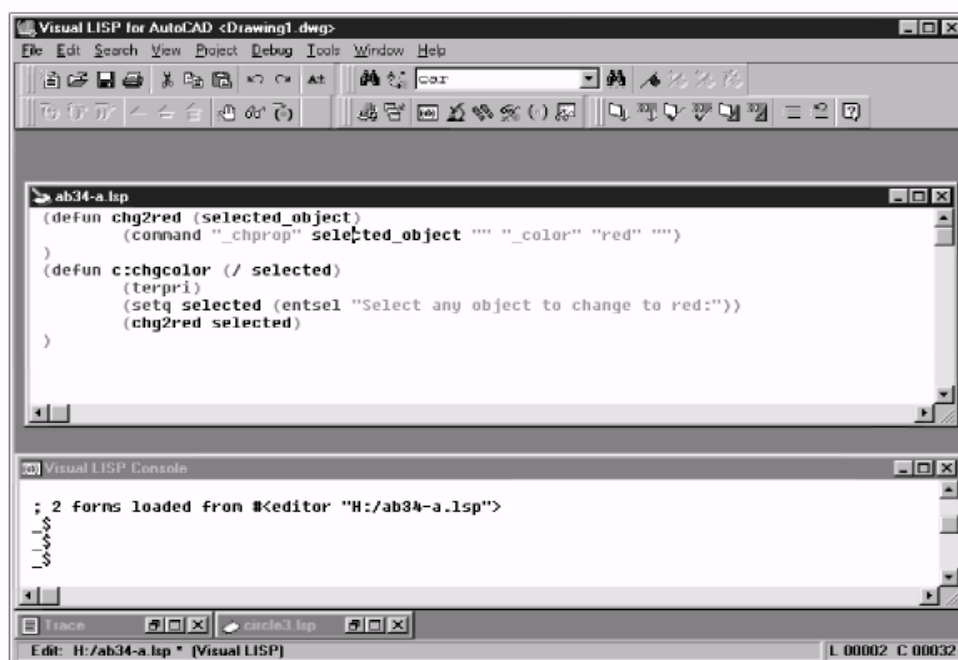
Рис 3. Файл AutoLISP, открытый в отдельном окне Visual LISP
