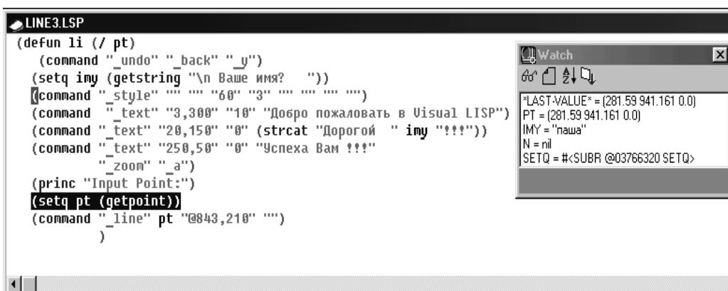
Рис. 7. Пошаговая отладка программы LI в текстовом окне Visual LISP с просмотром значений переменных в окне наблюдений
