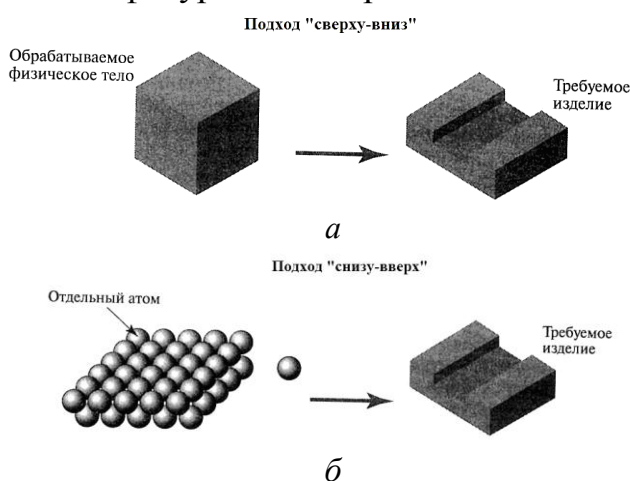
Рисунок 1.5 – Подходы наномонтажа для получения требуемого изделия: а – «сверху-вниз» с последовательным уменьшением размеров до требуемых; б – «снизу-вверх» путем сборки на атомарном уровне
