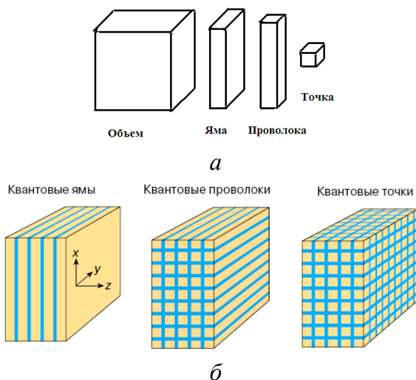
Рисунок 1.12 – Последовательность прямоугольных наноструктур (а) и геометрические области квантования в квантоворазмерных структурах (б)
