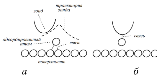
Рисунок 1.7 – Иллюстрация траектории острия зонда СТМ над адсорбированным на поверхности материала атомом:
