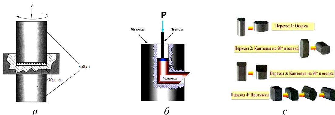
Рисунок 1.28 – Основные методы ИПД:
