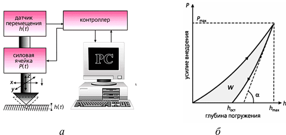
Рисунок 1.4 – Принципиальная схема нанотестирования поверхности (а) и типичная диаграмма «сила-перемещение» при наноиндентировании – аналог диаграммы \sigma - \epsilon в традиционных макроиспытаниях (б): h_{max} – максимальная глубина внедрения индентора; h_{ост} – глубина отпечатка, оставшегося после снятия нагрузки; W – поглощенная энергия
