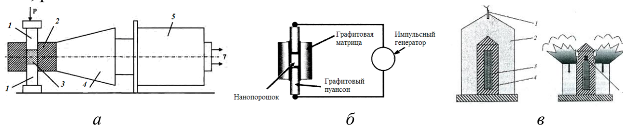
Рисунок 1.27 – Схемы методов динамического прессования:
