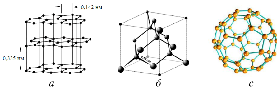
Рисунок 1.23 – Кристаллическая решетка графита (а); алмаза (б); молекула фуллерена (в)
