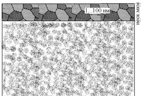
Рисунок 1.29 – Нанокристаллическое покрытие
