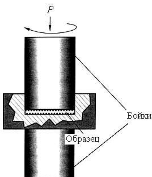
Рисунок 7.4 – Схема метода кручения под давлением
