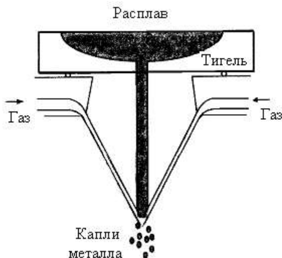
Рисунок 7.11– Схема установки для получения капель металлических наночастиц газовой атомизацией
