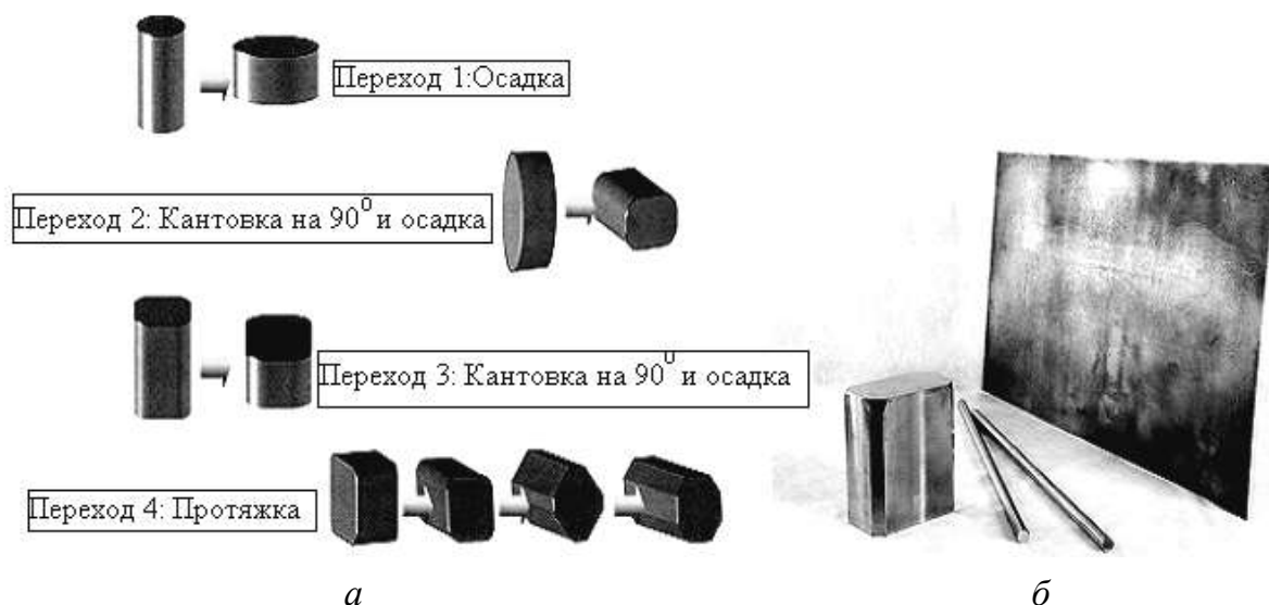
Рисунок 7.6 – Схема всесторонней ковки (а) и наноструктурные полуфабрикаты из титанового сплава ВТ6 (б), полученные данным методом
