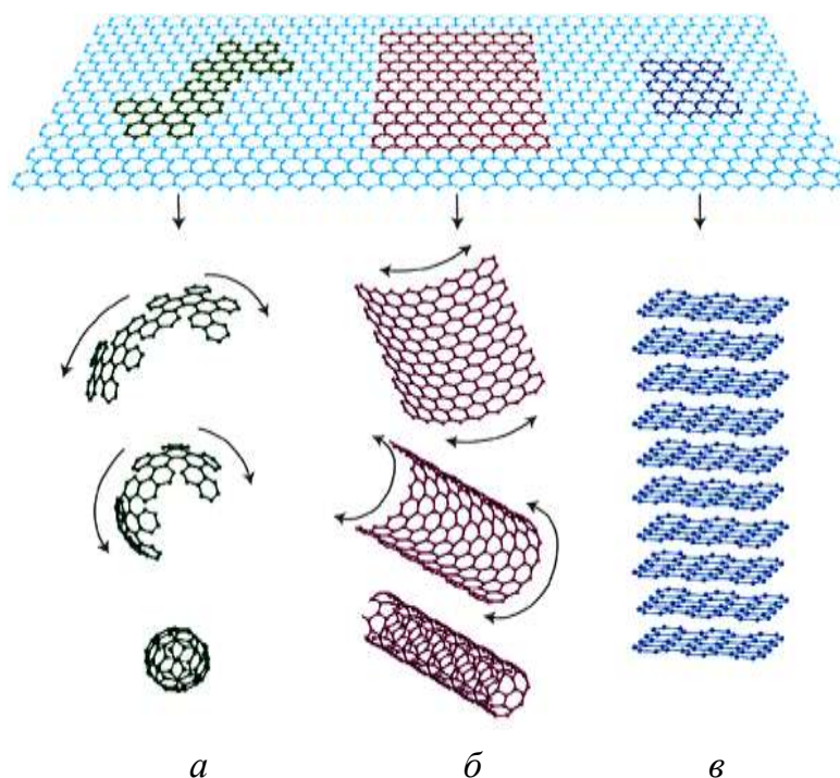
Рисунок 6.22 – Графен как строительный материал для других аллотропных модификаций углерода
