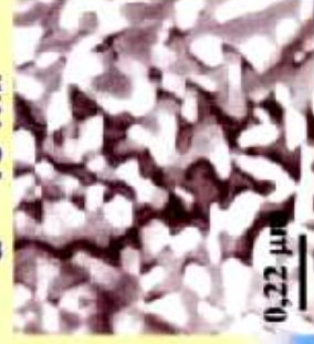
Рисунок 10.5 – Создание тонкопленочных наноструктур для термоэлектрических преобразователей энергии
