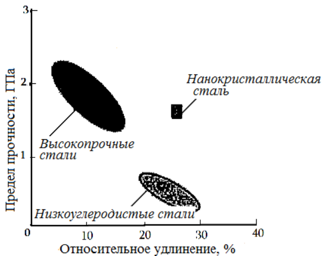
Рисунок 4.11 – Соотношение между прочностью и пластичностью для сталей
