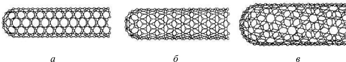
Рисунок 6.12 – Примеры некоторых возможных структур углеродных нанотрубок, зависящих от способа сворачивания графитового листа: a – кресельная структура; б – зигзагообразная структура, в – хиральная (спиралевидная) структура
