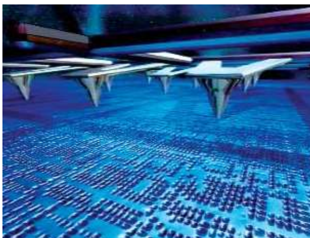
Рисунок 2.11 – Считывание информации с жесткого диска с помощью матрицы кантилеверов (« Millipede »)
