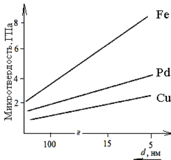
Рисунок 4.9 – Влияние размера зерна на микротвердость материалов
