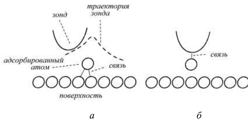
Рисунок 3.4 – Иллюстрация траектории острого зонда СТМ над адсорбированным на поверхности материала атомом:
