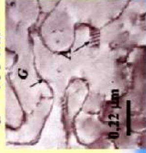
Рисунок 10.5 – Создание тонкопленочных наноструктур для термоэлектрических преобразователей энергии
