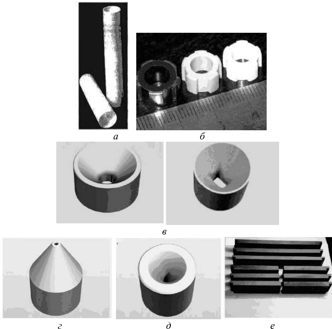
Рисунок 8.3 – Керамические изделия с наноструктурой, полученные компактированием нанопорошков:
