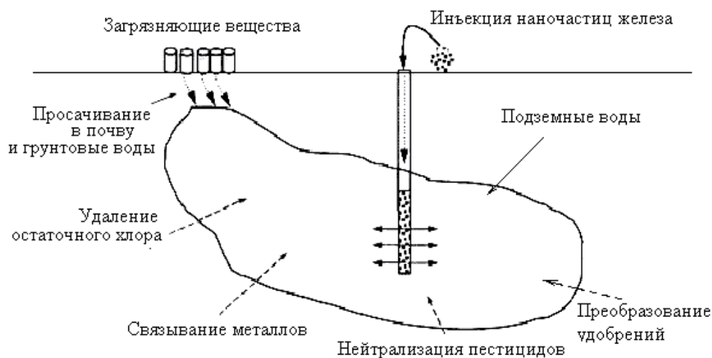
Рисунок 8.17 – Схема очистки почвы наночастицами железа
