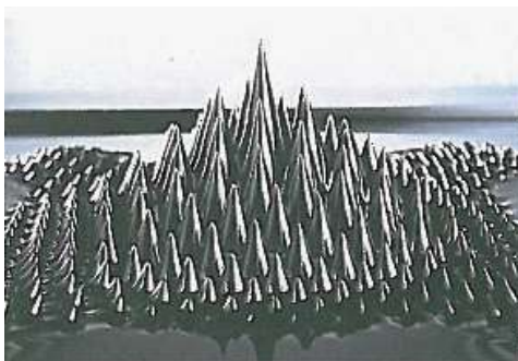
Рисунок 8.5 – Магнитная жидкость, помещенная в магнитное поле
