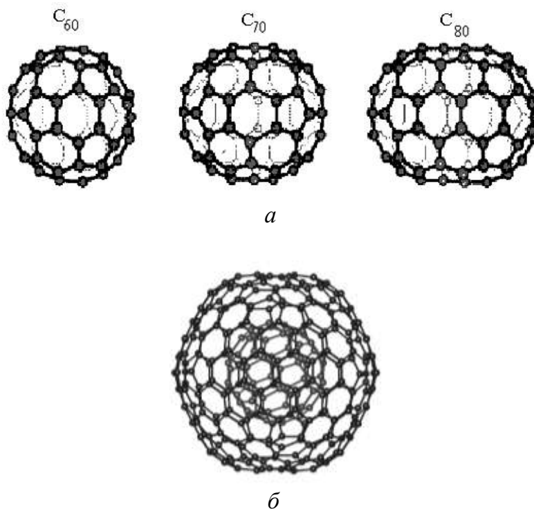
Рисунок 6.3 –Примеры структур на основе углеродных кластеров: а – фуллерены C 60 , C 70 , C 80 ; б – многослойный фуллерен C 60 /C 240
