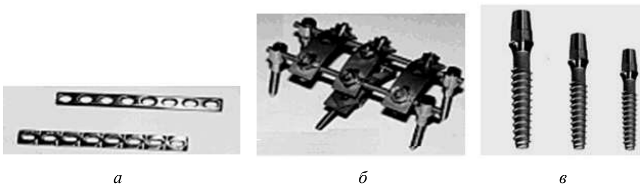
Рисунок 7.9 – Медицинские имплантаты, изготовленные из наноструктурного титана:
