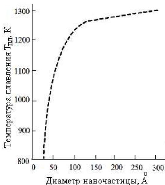
Рисунок 4.7 – Зависимость температуры плавления наночастиц золота от размера зерна
