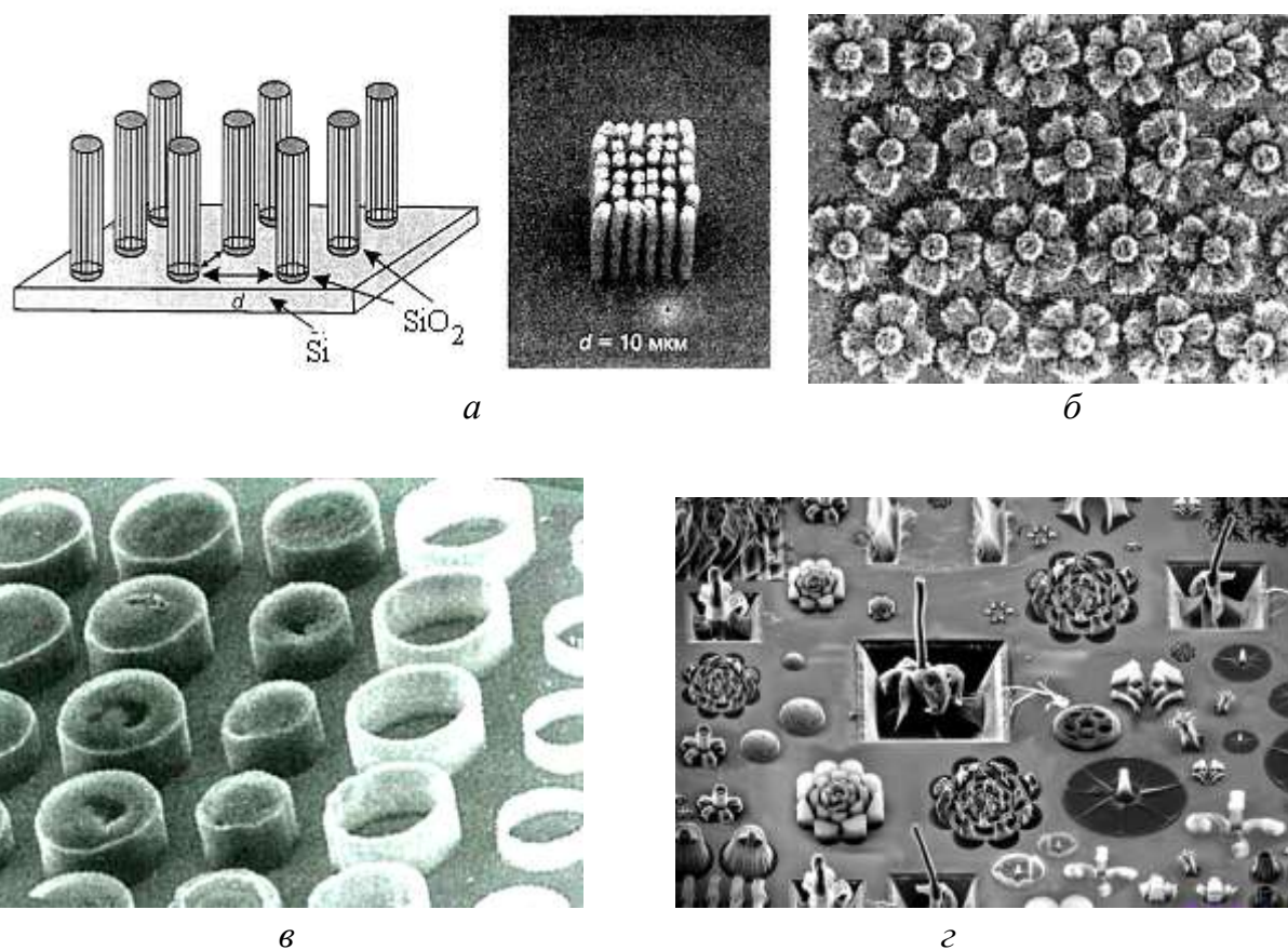
Рисунок 6.16 – Управляемый рост упорядоченных массивов нанотрубок: а – схема получения колонн из вертикально упорядоченных нанотрубок; б – вертикальные (в центре) и горизонтальные ориентированные нанотрубки; в – искусственно выращенная решетка из многослойных углеродных нанотрубок; г – массив выращенных нанотрубок для создания микросхем
