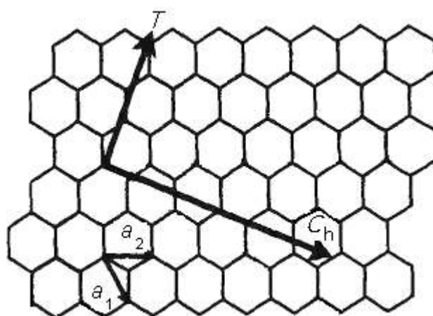
Рисунок 6.11 – Возможные ориентационные направления сворачивания графитового листа при образовании нанотрубок различной структуры:
