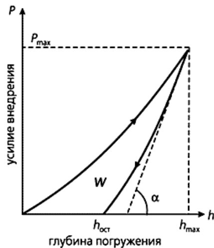
Рисунок 2.19 – Типичная диаграмма «сила-перемещение» при наноиндентировании (аналог диаграммы \sigma - \varepsilon в традиционных макроиспытаниях):
