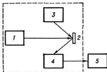
Рисунок 2.13 – Блок-схема электронного оже-спектрометра:
