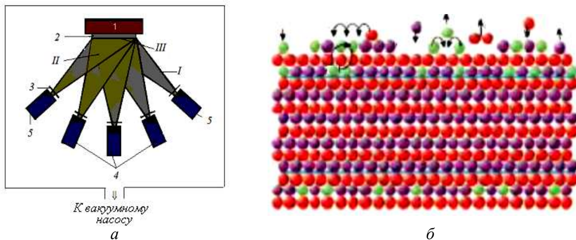
Рисунок 3.14 – Схема установки молекулярно-лучевой эпитаксии (а) и схема роста пленки путем «атомной укладки» (б):
