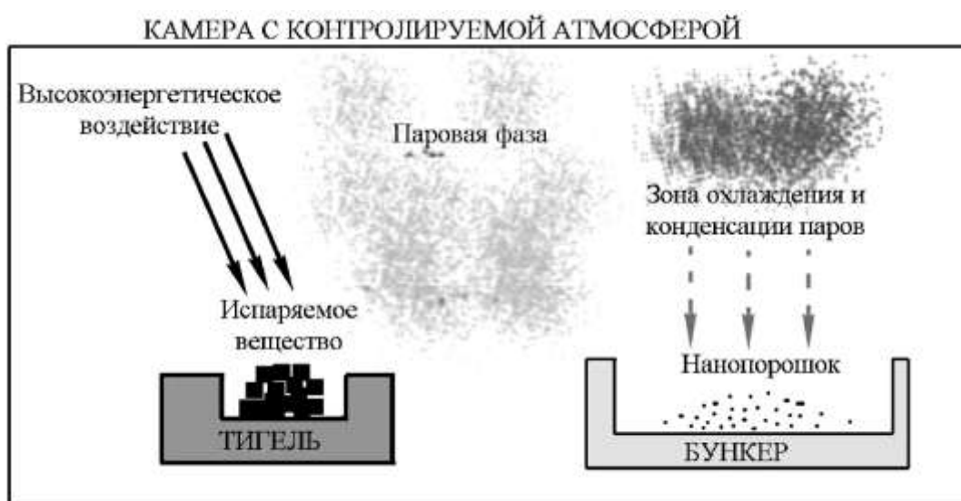
Рисунок 5.3 - Принципиальная схема получения нанопорошков методом термического испарения и конденсации материала из паровой фазы
