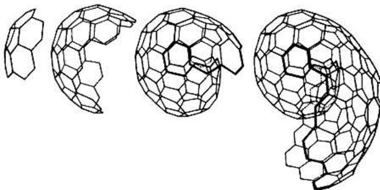
Рисунок 6.5 – Механизм формирования фуллерена
