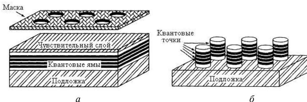
Рисунок 3.20 – Формирование массива квантовых точек методом литографии:
