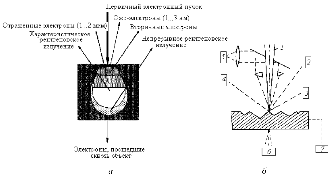
Рисунок 2.2 – Виды излучений, формирующихся при взаимодействии электронов с поверхностью материала (а) и схема регистрации информации об объекте в сканирующем электронном микроскопе (б):
