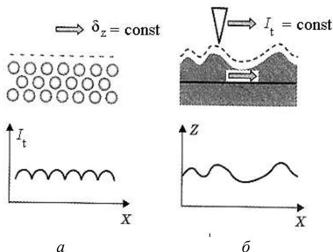
Рисунок 2.7 – Принципы формирования изображения в СТМ в режиме постоянного расстояния от зонда до поверхности (а) и в режиме постоянного туннельного тока (б)
