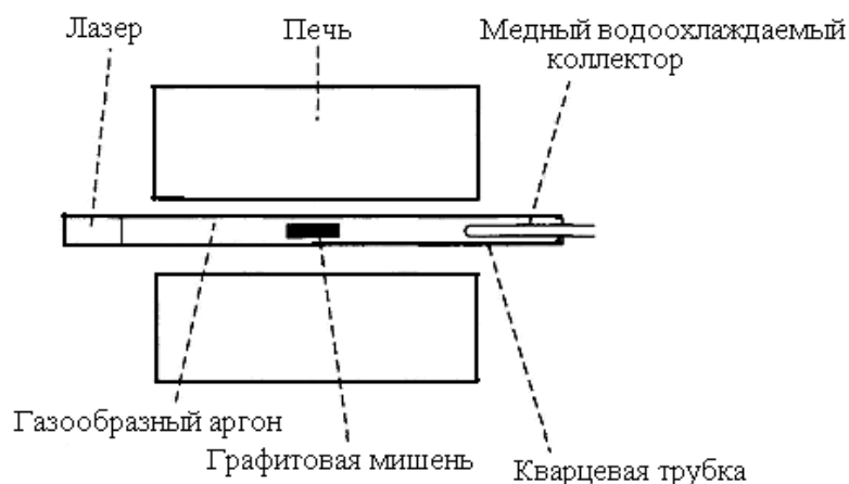
Рисунок 6.14 – Установка для синтеза углеродных нанотрубок лазерным испарением
