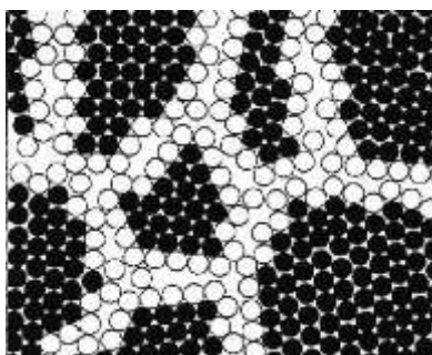
Рисунок 4.3 – Модель строения нанокристаллического материала
