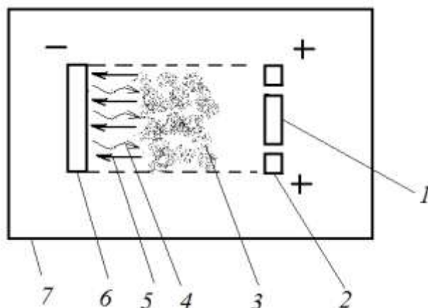
Рисунок 7.14 – Упрощенная схема установки катодного распыления
