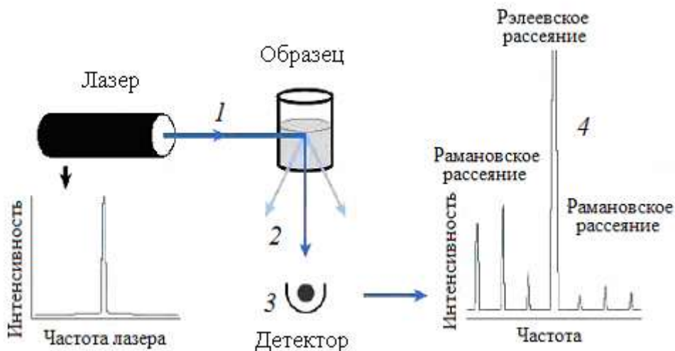
Рисунок 2.14 – Схема исследования с помощью рамановской спектроскопии:
