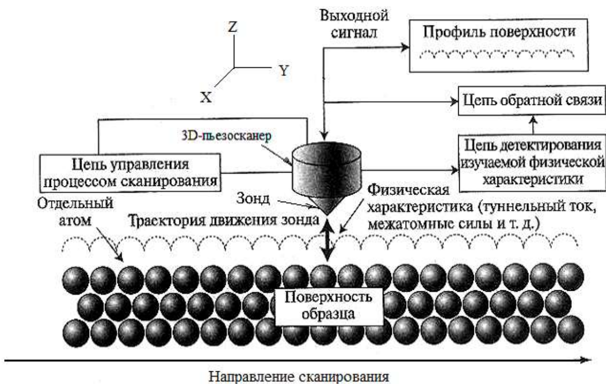
Рисунок 2.5 – Типовая схема зондовых сканирующих микроскопов
