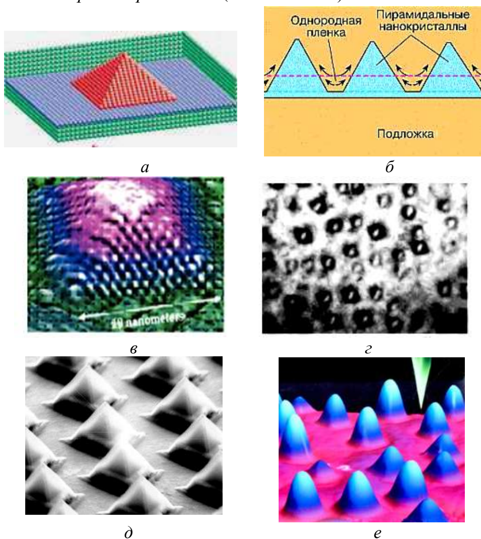
Рис. 3.16 – Квантовые точки: a – модель квантовой точки; б – формирование квантовых точек методом МЛЭ;
