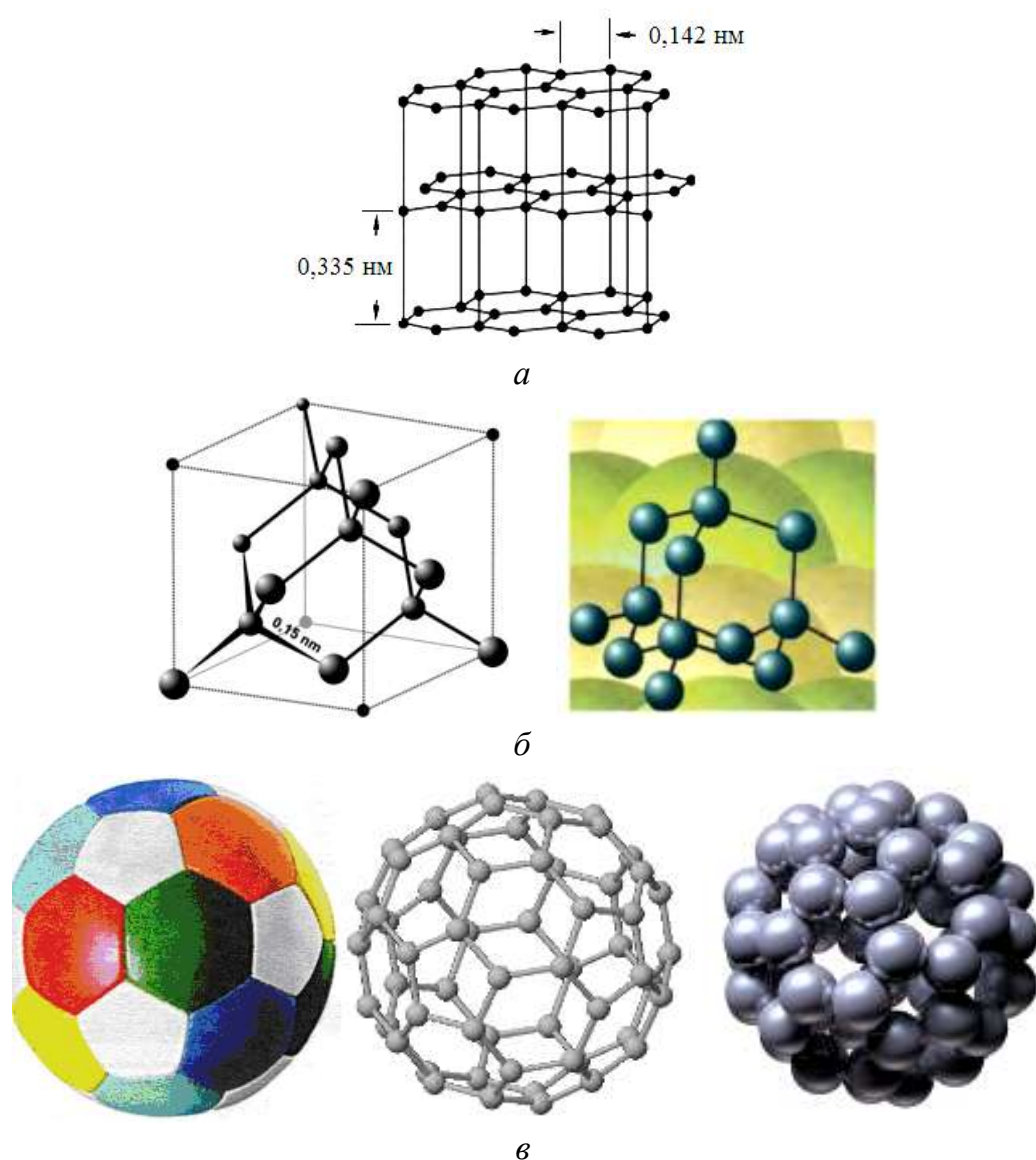
Рисунок 6.2 – Кристаллическая решетка графита ( a ); алмаза ( б ); молекула фуллерена (аналогия с футбольным мячом) ( в )
