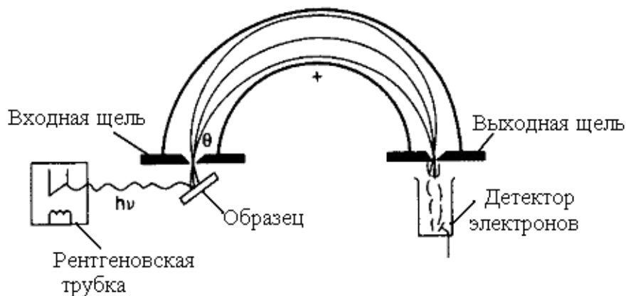
Рисунок 2.15 – Схема рентгеновского фотоэлектронного спектрометра
