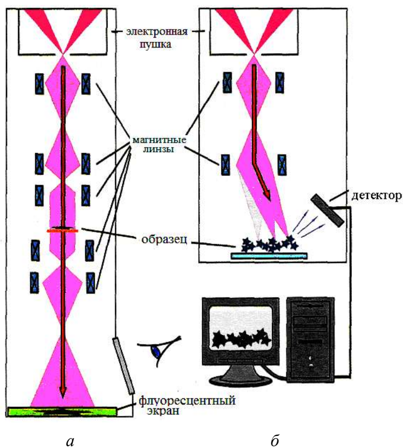
Рисунок 2.3 – Принцип работы электронного просвечивающего (а) и сканирующего (б) микроскопов
