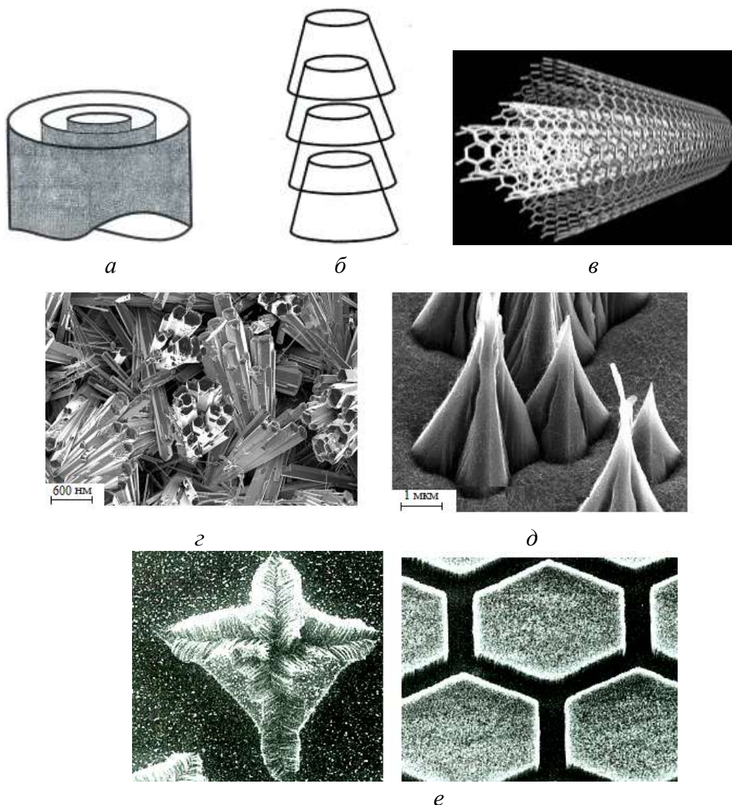
Рисунок 6.13 – Примеры структур на основе углеродных нанотрубок: a, б – схемы многослойных цилиндрических и конических нанотрубок соответственно; в – многослойная нанотрубка C_{60}/C_{240}/C_{540} ; г – «колонии» углеродных нанотрубок; д – «связки» углеродных нанотрубок на поверхности кремния; е – примеры нанотрубок, искусственно (каталитически) выращенных в специальных шаблонах
