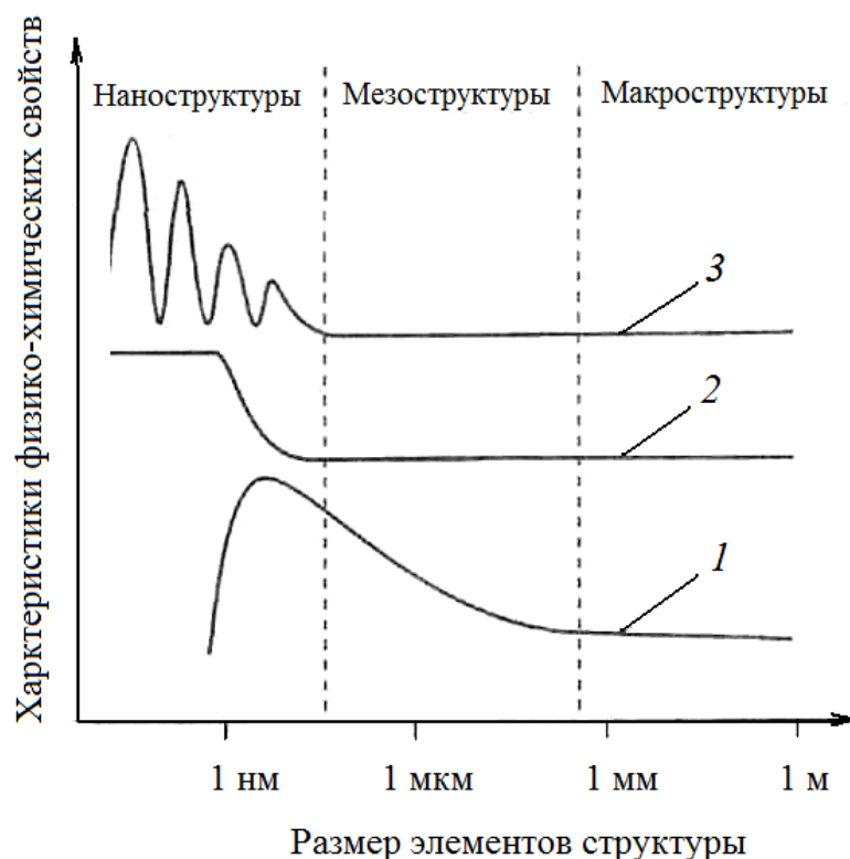
Рисунок 4.1 – Изменение физико-химических характеристик материала в зависимости от размера структуры:
