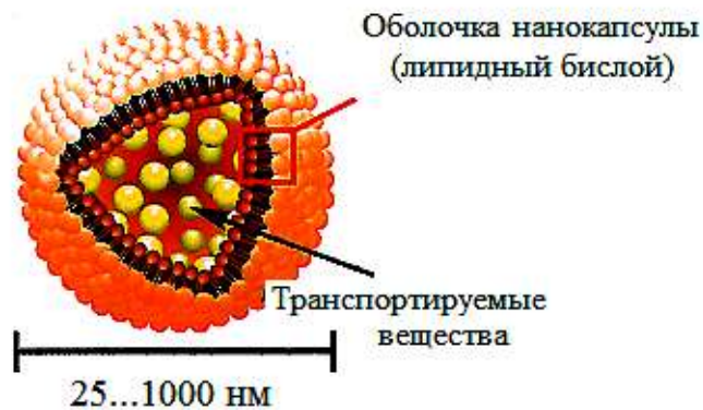
Рисунок 8.14 – Структура «наноконтейнера»
