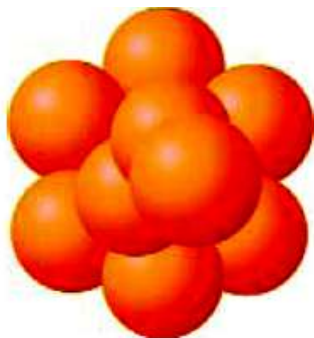
Рисунок 3.11 – Наночастица из 16-ти атомов аргона
