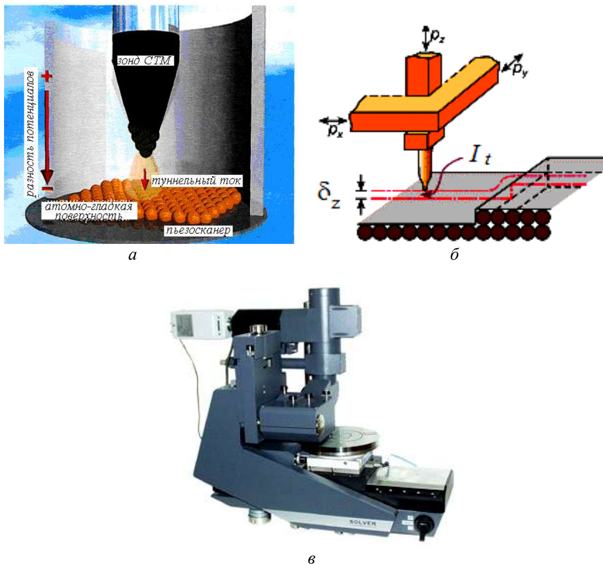
Рисунок 2.6 – Принцип реализации сканирующей туннельной микроскопии: а – общая схема работы СТМ; б - принцип действия СТМ:
