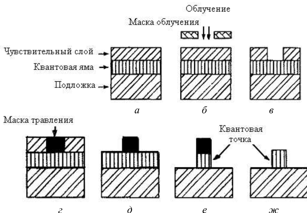
Рисунок 3.19 – Этапы формирования квантовой точки (или проволоки) методом электронно-лучевой литографии
