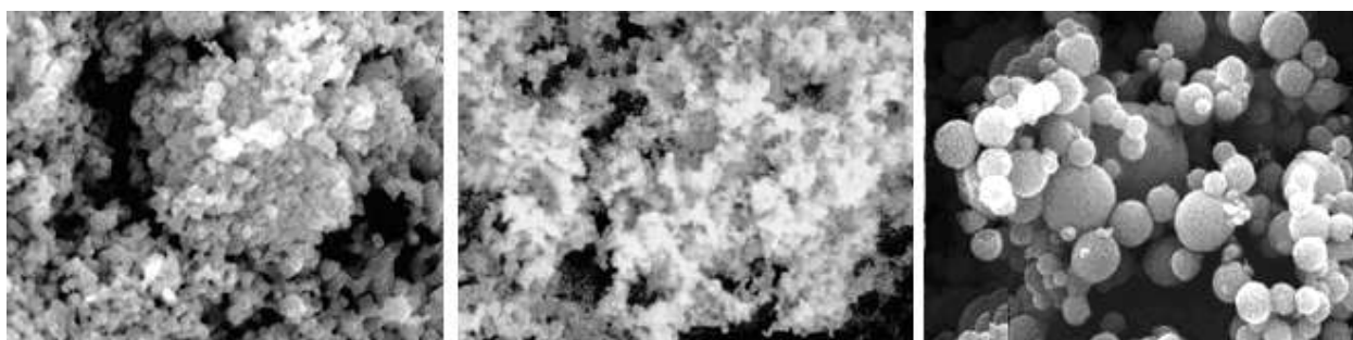
Рисунок 5.4 – Нанопорошки, полученные различными физическими методами: а - карбид вольфрама (средний размер частиц ~ 30 нм), плазмохимический метод; б - карбид титана (средний размер частиц ~ 10 нм), плазмохимический метод; в - нанопорошок алюминия (средний размер частиц ~ 30...100 нм), метод ЭВП
