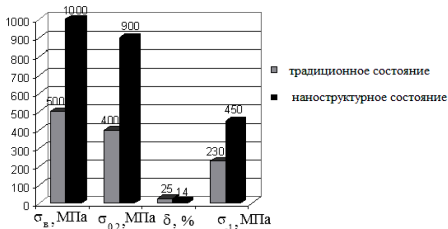
Рисунок 4.10 – Механические свойства технического чистого титана с традиционной структурой и в наносостоянии
