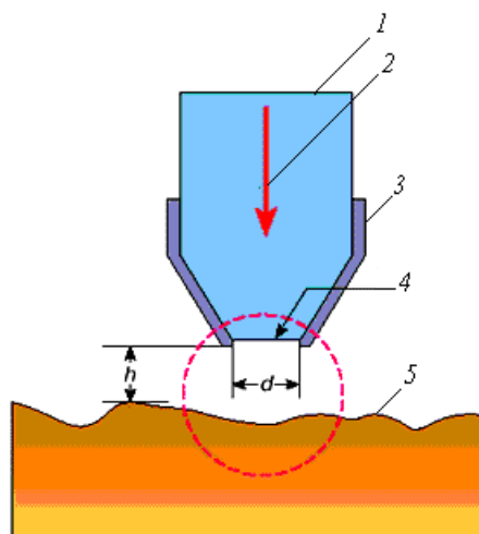
Рисунок 2.9 – Схема формирования сигнала в СОМБП:
