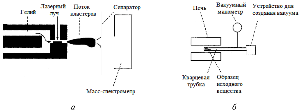
Рисунок 3.13 – Схемы установок для получения металлических атомных кластеров:
