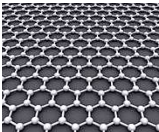
Рисунок 6.21 – Структура графена (расстояние между атомами 0,142 нм)
