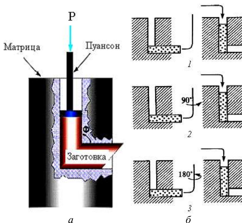
Рисунок 7.5 – Схема равноканального углового прессования (а) и возможные варианты равноканального углового прессования (б): 1 – неизменная ориентация заготовки; 2 – поворот заготовки на 90^\circ ; 3 – поворот заготовки на 180^\circ
