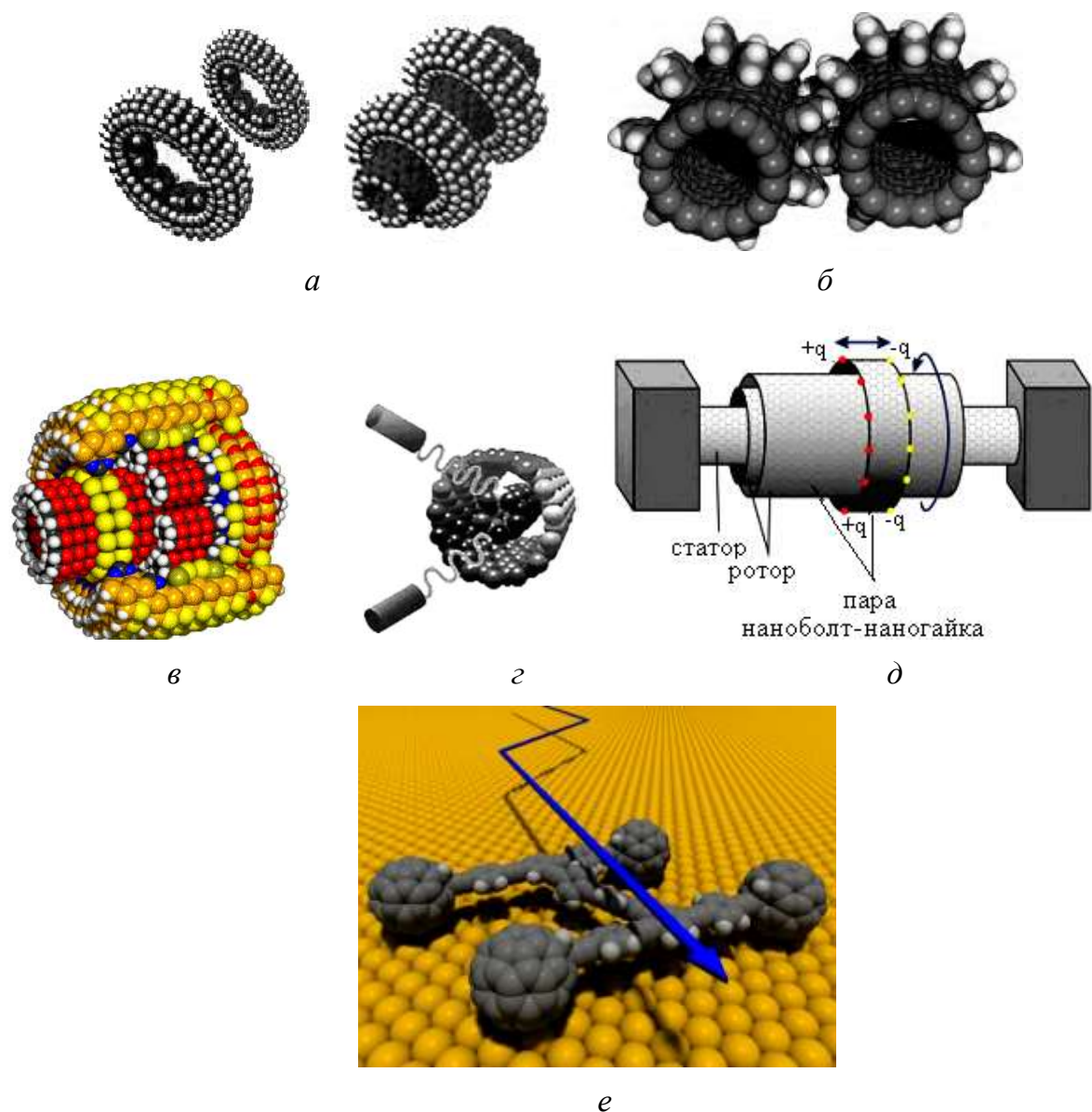
Рисунок 8.11 – Некоторые примеры НЭМС на основе наноматериалов: a – наноподшипники; б – наношестеренки на основе углеродных нанотрубок; в – молекулярный редуктор; г – наномотор, приводимый в движение светом; д – принципиальная схема наномотора (заряды на краях слоев могут быть получены химической адсорбцией и служить для управления наномотором с помощью электрического поля); е – «наноавтомобиль» из 300 атомов с колесами из молекул фуллерена, связанных химическими связями с «каркасом», ширина автомобиля \sim 4 нм
