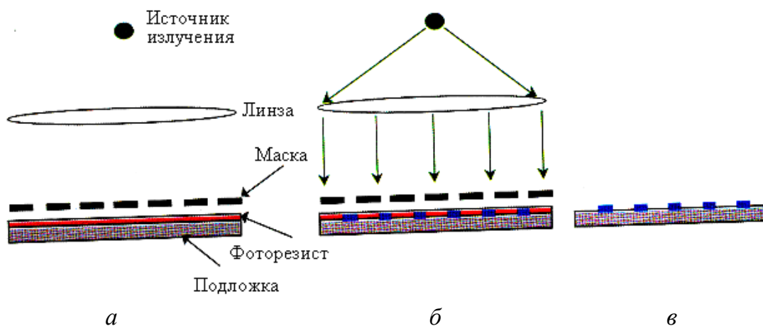
Рисунок 3.18 – Принципиальная схема литографии
