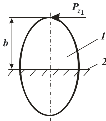
1 – зерно; 2 – уровень связки круга
