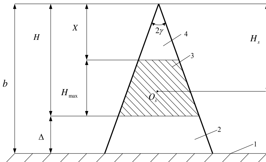
1 – связка, 2 – зерно, 3 – сечение среза, 4 – изношенная часть зерна, O_s – геометрический центр тяжести сечения среза
