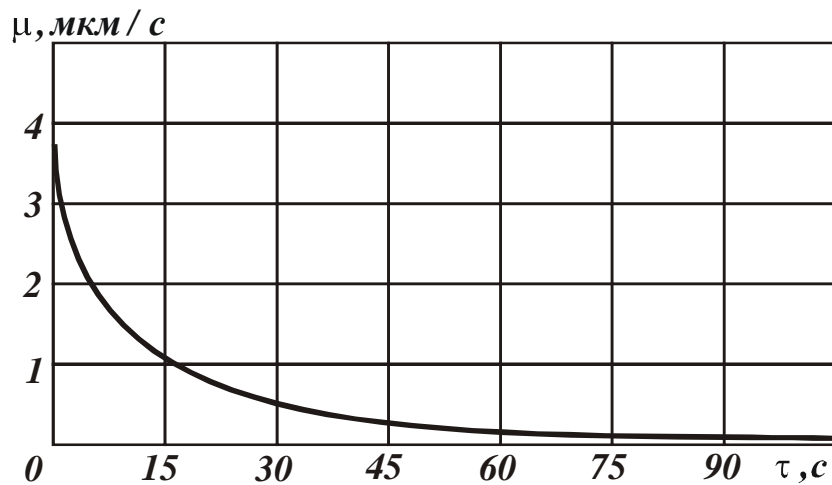
Рис. 4.14. Влияние продолжительности обработки \tau на скорость снижения высоты зерен \mu в переходной фазе шлифования синтетического сверхтвёрдого материала АСПК: V_{кр} = 20 м/с; P_n = 3,0 МПа [61]
