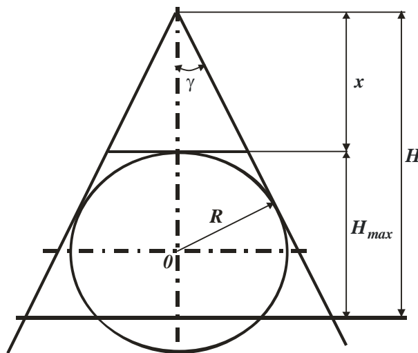
Рис. 3.3. Расчетная схема
