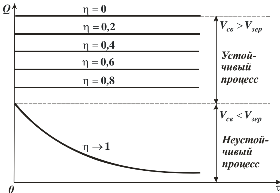
Рис. 4.23. Характер изменения производительности обработки Q с течением времени шлифования \tau для различных значений безразмерного коэффициента \eta
