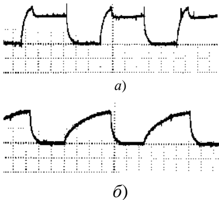
Рисунок 4 – Осциллограмма тока
