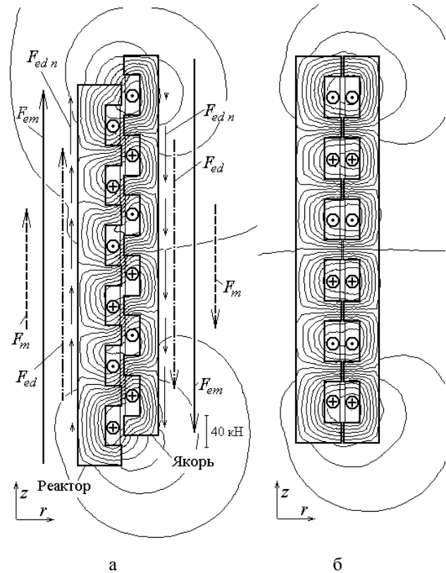
Рис.2. Симметричные половины сечения магнитной системы ЛИЭД с вариантами расположения реактора: а – исходное положение; б – конечное положение
