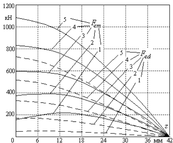
Рис.4. Изменение результирующих сил F_{em} и F_{ed} при различных положениях реактора ( z=0 – исходное по рис.2,а; z=42 мм – конечное по рис.2,б) и при разных значениях МДС F_{En} : 1 – 20 кА; 2 – 40 кА; 3 – 60 кА; 4 – 80 кА; 5 – 100 кА
