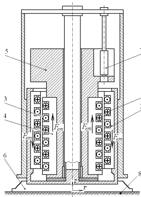
Рис.1. Устройство линейного электродвигателя: 1 – обмотка якоря; 2 – магнитопровод якоря; 3 – обмотка реактора; 4 – магнитопровод реактора; 5 – инертная масса; 6 – опорная плита-конус; 7 – амортизатор; 8 – грунт
