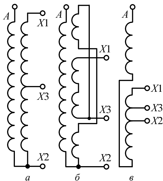
Рисунок 6.1 – Схеми виконання регулювальних відгалужень обмотки вищої напруги
