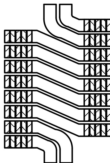
Рисунок 5.6 – Гвинтова обмотка з радіальними охолодними каналами
