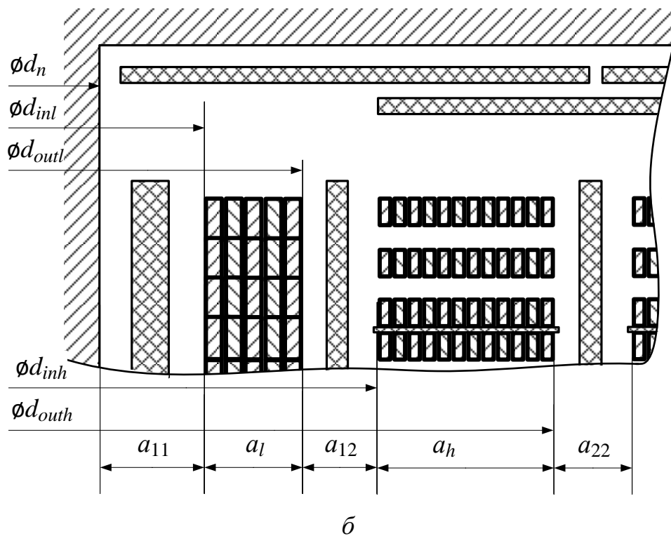
Рисунок 6.5 – Розміри обмоток трансформатора:
