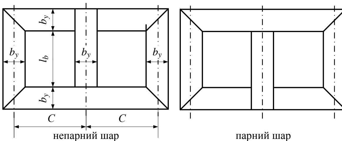
Рисунок 8.2 – Розміри та схема шихтування магнітної системи трансформатора
