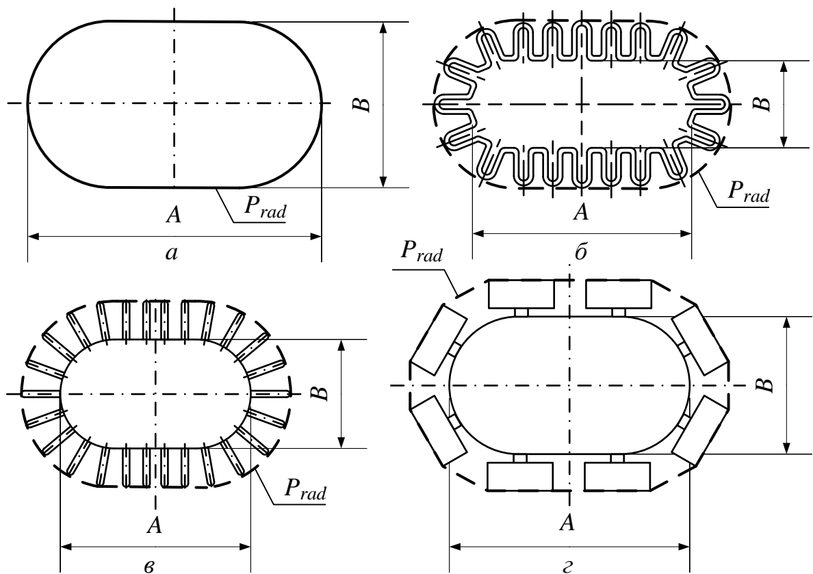
Рисунок 12.6 – Периметр поверхні тепловіддачі, яка здійснюється випромінюванням: a – для гладкого бака; б – для хвилястого бака; в – для трубчастого бака; г – для бака з навісними радіаторами над температурою зовнішнього повітря, °С,
