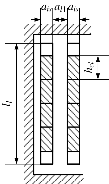
Рисунок 5.3 – Розміри циліндричної обмотки з осьовим каналом
