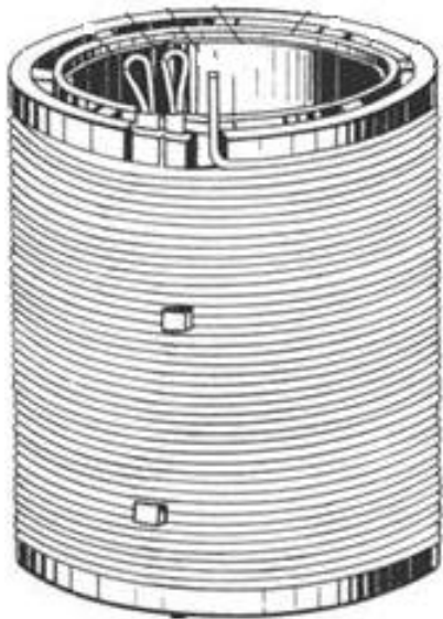
Рисунок 6.2 – Циліндрична багат шарова обмотка з осьовим каналом
