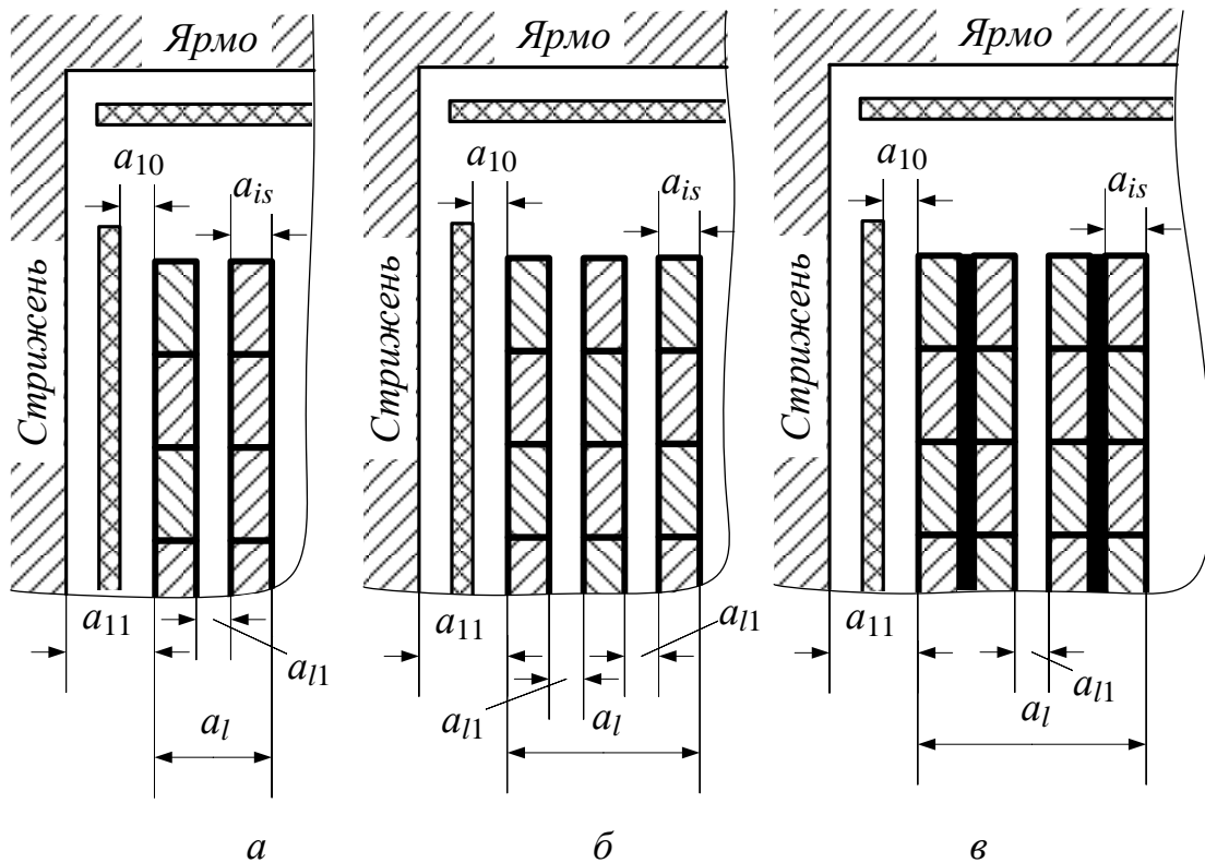
Рисунок 5.4 – Радіальні розміри циліндричної обмотки з проводу прямокутного перерізу:
