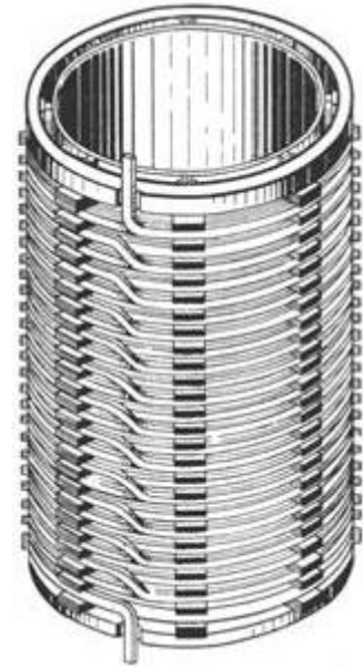
Рисунок 6.4 – Спіральна безперервна катушкова обмотка з проводу прямокутного перерізу
