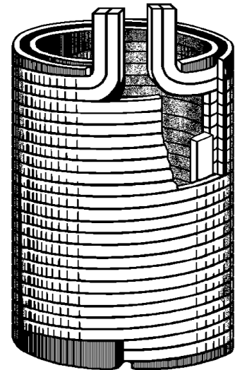
Рисунок 5.1 – Циліндрична двошарова обмотка з осьовим каналом з проводу прямокутного перерізу
