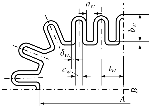
Рисунок 12.2 – Розміри елементів бака із хвилястими стінками
