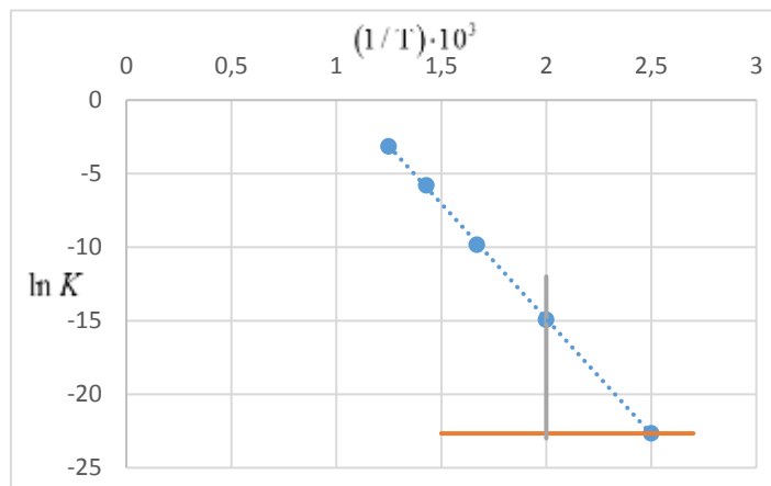
Залежність \ln K^0 = f(1/T)
