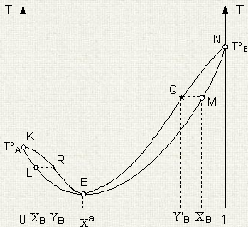
(А) Состав, мольн. доля В
