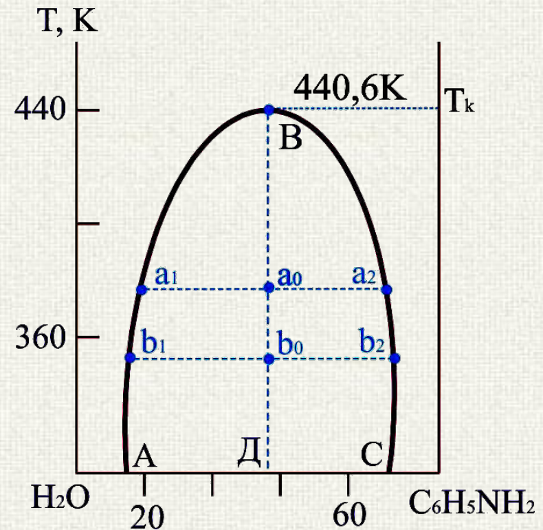
Діаграма стану системи «вода-анілін» з верхньою критичною температурою розшарування
