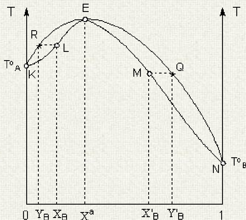
(Б) Состав, мольн. доля В
