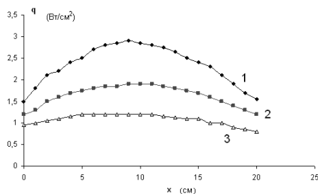
Рис.1. Распределения плотности энергии нагревателя поплддя расстояния , 1 – 20 (см), 2 – 30 (см), 3 – 40 (см).
