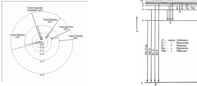
Рис.2 Стационарные орбиты атома водорода и образование спектральных серий.
