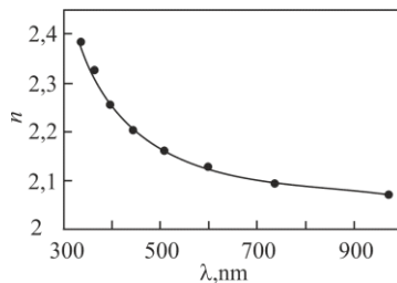
Рис. 2. Спектральная зависимость показателя преломления n(\lambda) тонких пленок KPb_2Cl_5 .
