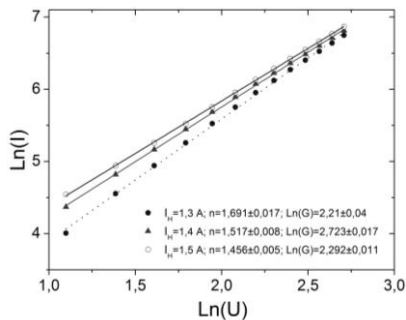
Рис. 5. Зависимость LnI(LnU) для различных токов накала катода.
