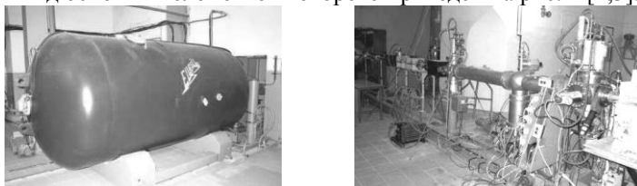
Рис.1. Внешний вид элементов электростатического ускорителя заряженных элементарных частиц типа «ELIAS» (НИЦ «ХФТИ», 2010)
