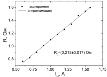
Рис. 7. Зависимость сопротивления нити от тока накала.
