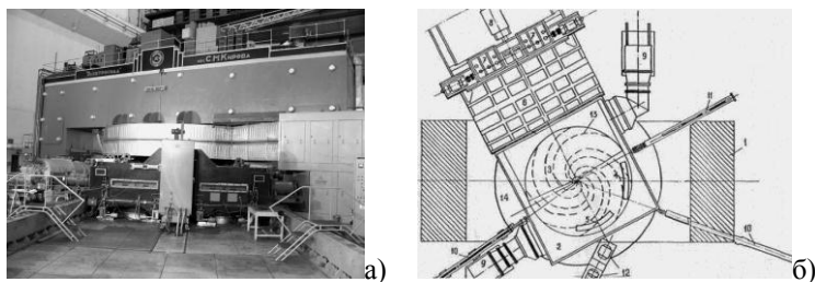
Рис. 3. а) фазотрон Лаборатории ядерных проблем ОИЯИ; б) Схема фазотрона Лаборатории ядерных проблем ОИЯИ.
