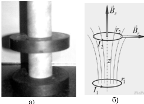
Рис. 1. Магнитный маятник: а) общий вид; б) конфигурация осесимметричного магнитного поля.
