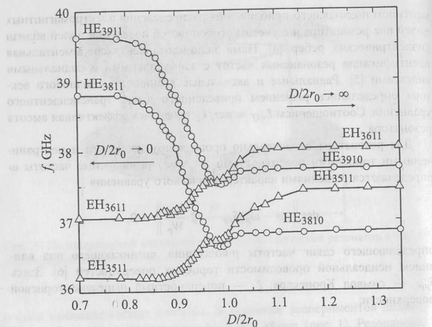
Рис. 2. Зависимость частот резонансных колебаний от приведенного радиуса.
