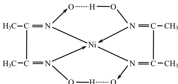
Рисунок 9.9. – Структурна формула диметилгліоксима (реактив Чугаєва)
