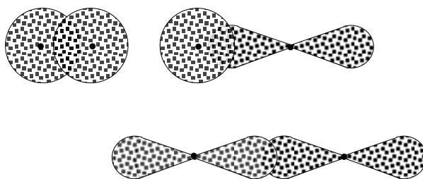
Рисунок 4.8 – Різновиди двохатомних молекул
