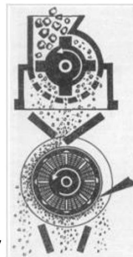
Схема магнітного сепаратору
