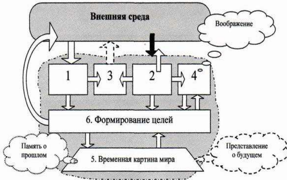
Рис. 18.1 Структура сознания.
