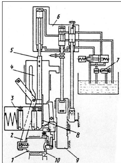
Рисунок 5.2 – Автоматичне використання фрез, що заокруглюють зубці
