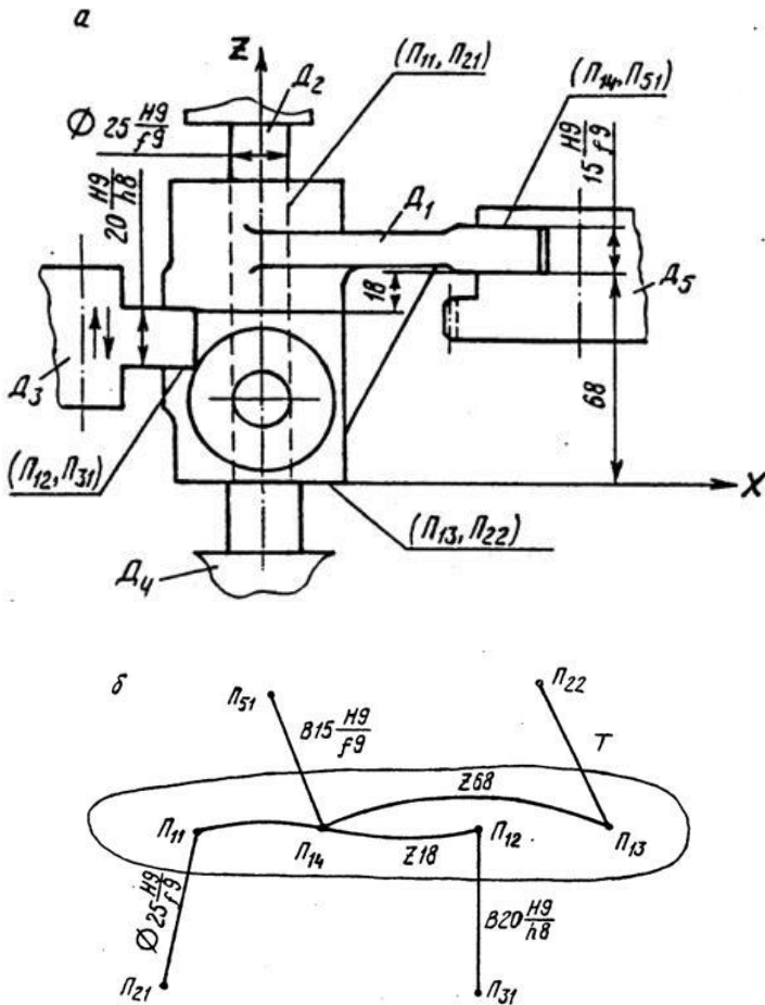
Рисунок 3.3 – Модель зв'язків деталі Д1 з іншими деталями вузла: а – схема механізму перемикаччя; б – граф зв'язків деталі Д1 з іншими деталями: П11 – П14 – поверхні з'єднань деталі Д1; П21, П31, П51 – поверхні з'єднань інших деталей (Д2, Д3, Д5)
