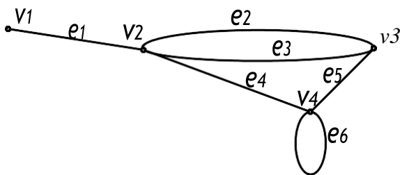
Рисунок 3.2 – Псевдограф
