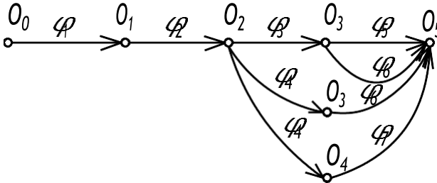
Рисунок 7.4 – Орграф
