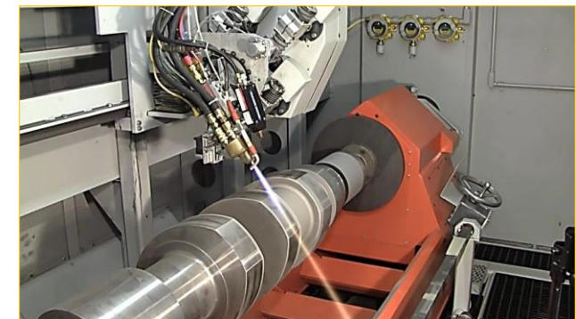
Плазмове напилення колінчастого валу
