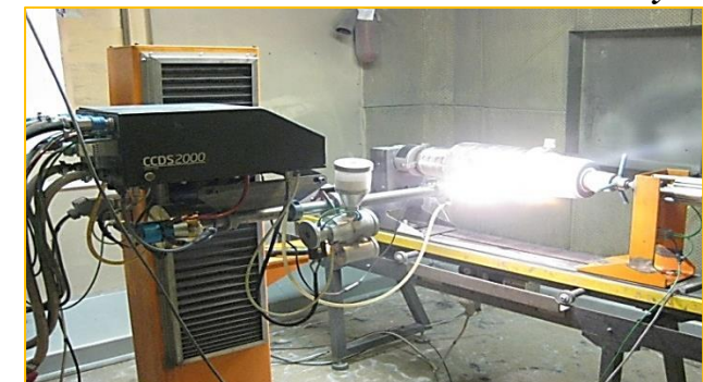
Детонаційне напилення валу
