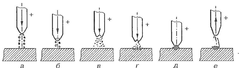
Рис. 5.1. Схема процесу електроіскрового легування
