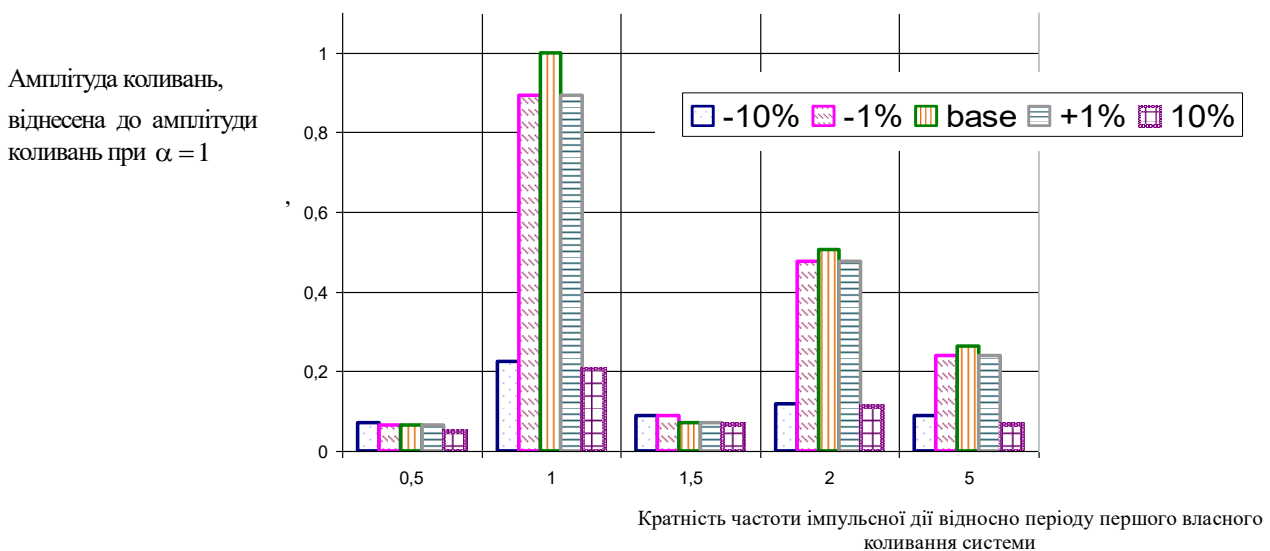
Рисунок 6 – Залежності амплітуд усталених коливань одномасової системи, віднесені до амплітуди при \alpha = 1 , при різних відлаштуваннях від резонансної частоти ( \pm 1\% , \pm 10\% )
