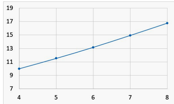
Рисунок 16 – Зміна 8-ї власної частоти від товщини панелей корпусу (Гц, мм)
