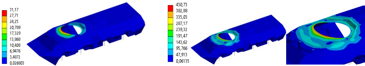
Картини розподілу еквівалентних напружень, МПа (час – середина пострілу)
