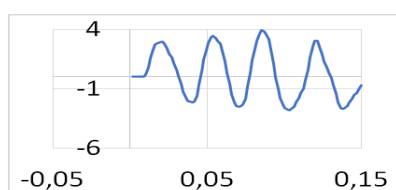
Рисунок 22 – Графік зміни кута коливань погонного кільця під час пострілу
