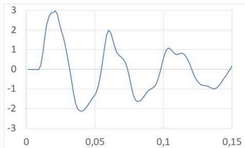
Рисунок 19 – Графік зміни кута коливань (градуси) погонного кільця під час пострілу (с)
