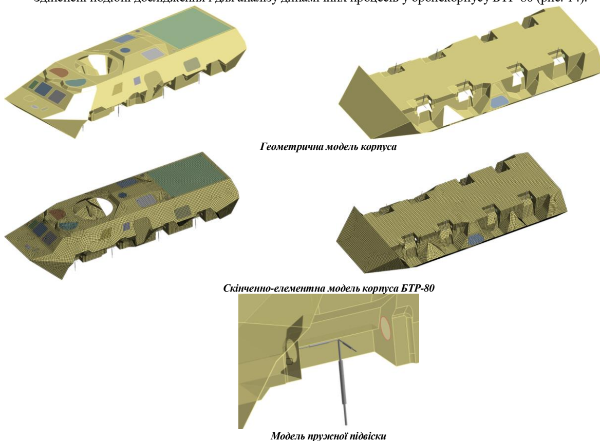
Рисунок 14 – Тестова модель бронекорпуса БТР-80 із однаковою товщиною панелей у різних проєкціях
