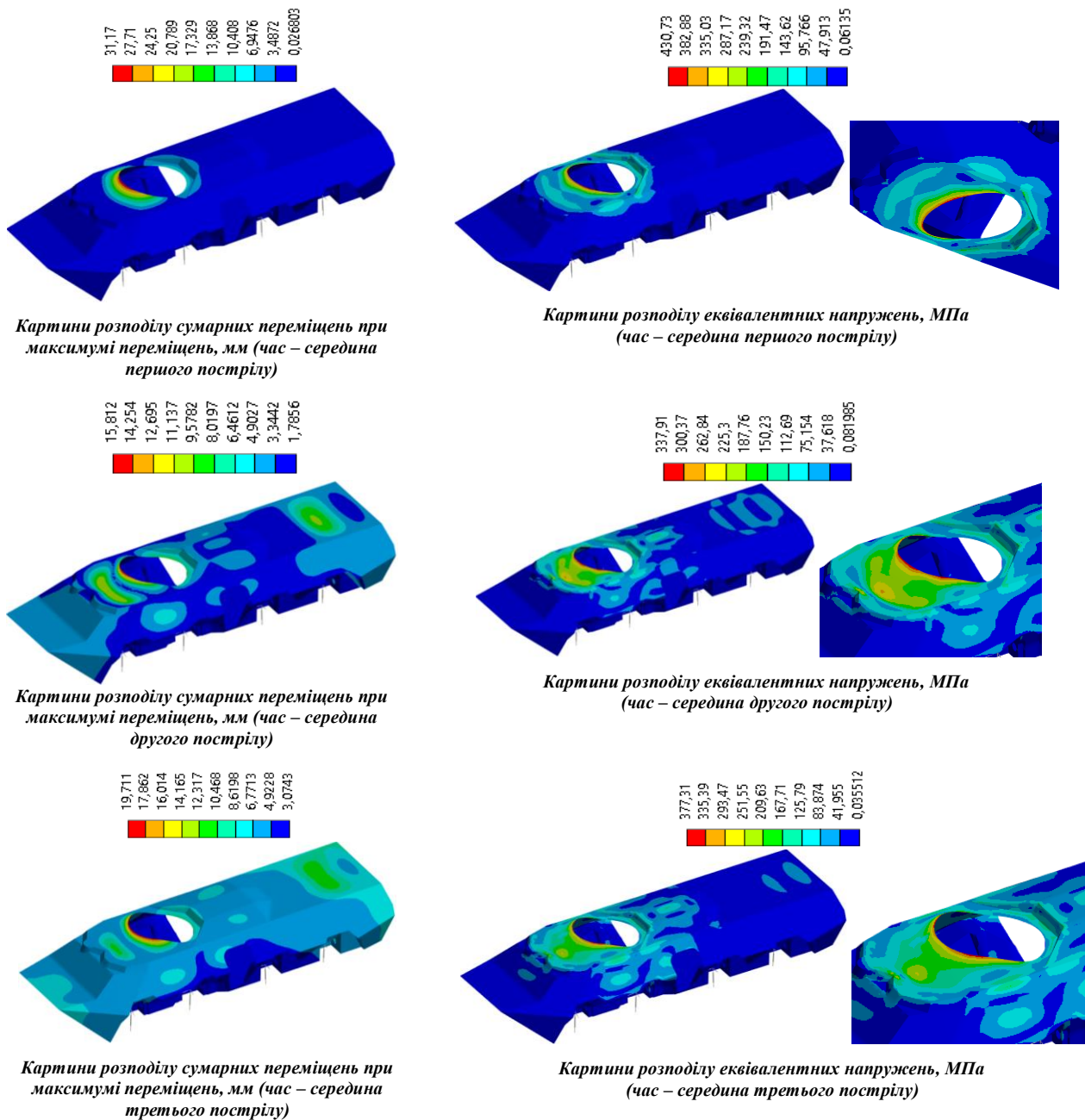
Рисунок 25 – Просторові розподіли характеристик напружено-деформованого стану броні корпусу БТР-80 (3 постріли)
