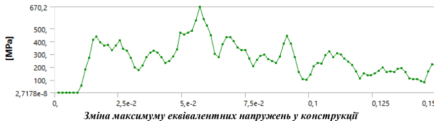
Рисунок 21 – Часові розподіли характеристик напружено-деформованого стану бронекорпусу БТР-80 (2 постріли)
