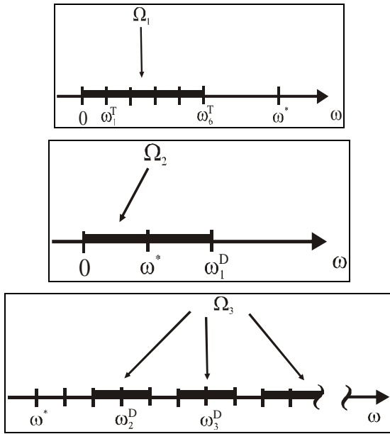
Рисунок 7 – До критеріїв відлаштування від резонансних режимів роботи вібромашини
