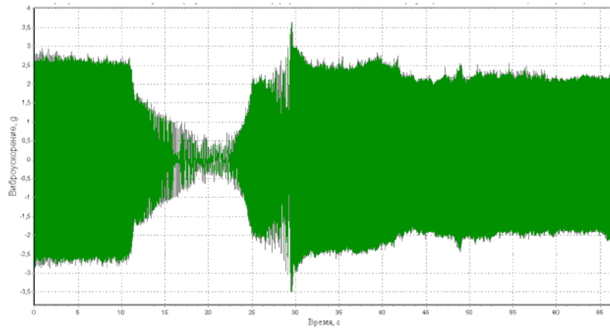
Рисунок 28 – Приклад віброграми (точка 1)
