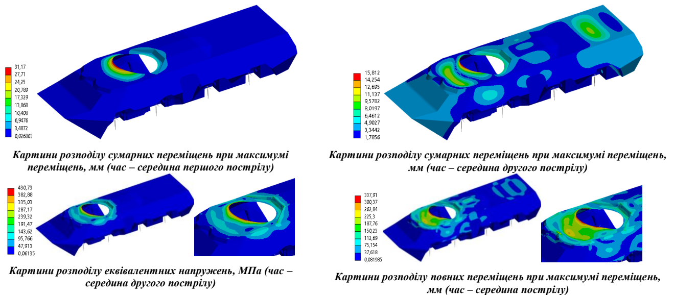
Рисунок 23 – Просторові розподіли характеристик напружено-деформованого стану броні корпусу БТР-80 (2 постріли)
