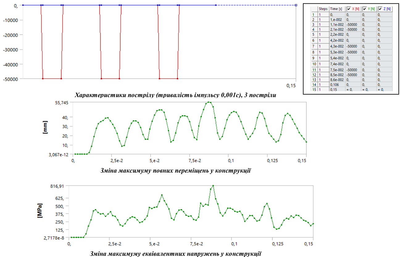
Рисунок 24 – Часові розподіли характеристик напружено-деформованого стану броні корпусу БТР-80 (3 постріли)
