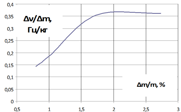
Рисунок 10 – Відносна зміна відлаштування спектру власних частот корпусу вібромашини від резонансів у діапазоні до 100 Гц \Delta^*/\Delta m від відносної величини зростання маси при різних схемах обрєбріння
