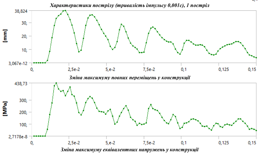
Рисунок 17 – Часові розподіли характеристик напружено-деформованого стану бронекорпусу БТР-80 (1 постріл)
