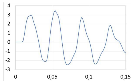
Рисунок 20 – Графік зміни кута коливань погонного кільця під час пострілу
