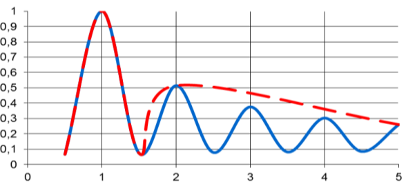
Рисунок 5 – Залежності амплітуд коливань ustalених від коефіцієнта повторності імпульсів, віднесених до амплітуди при \alpha = 1
