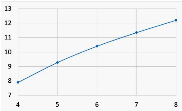
Рисунок 15 – Зміна 7-ї власної частоти від товщини панелей корпусу (Гц, мм)
