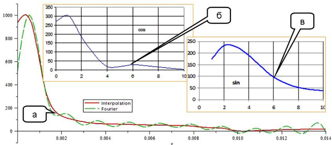
Рисунок 2 – Розподіл сили ударно-імпульсної взаємодії F_{\text{имп}}(t) (кН) між вибивною машиною і технологічним вантажем на інтервали ненульового значення (15 мс) та її подання у вигляді частинної суми ряду Фур'є (див. формулу (1)):
