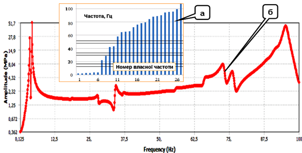
Рисунок 13 – Спектр власних частот коливань корпусу удосконаленої вибивної машини, отриманого з урахуванням рекомендацій за результатами ітераційного уточнення параметрів (а) та його амплітудно-частотна характеристика (б)
